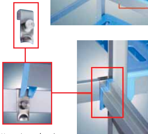
Montaje en ángulo
